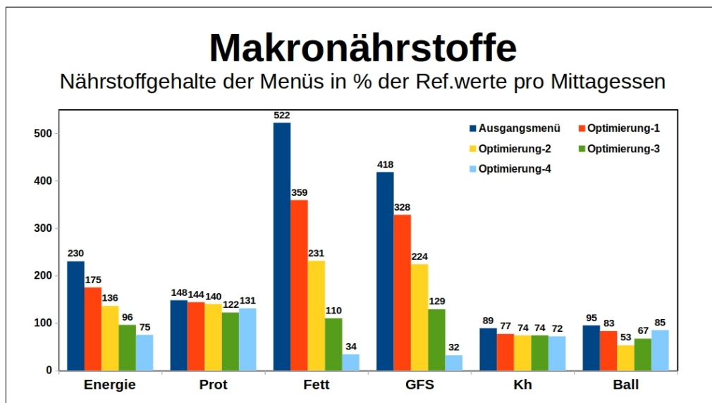
Abb. 6.1: Gehalt an Makronährstoffen
