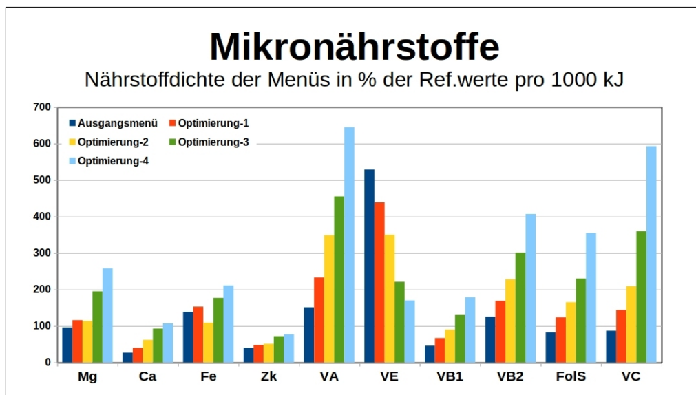
Abb. 6.3: Gehalt an Mikronährstoffen
