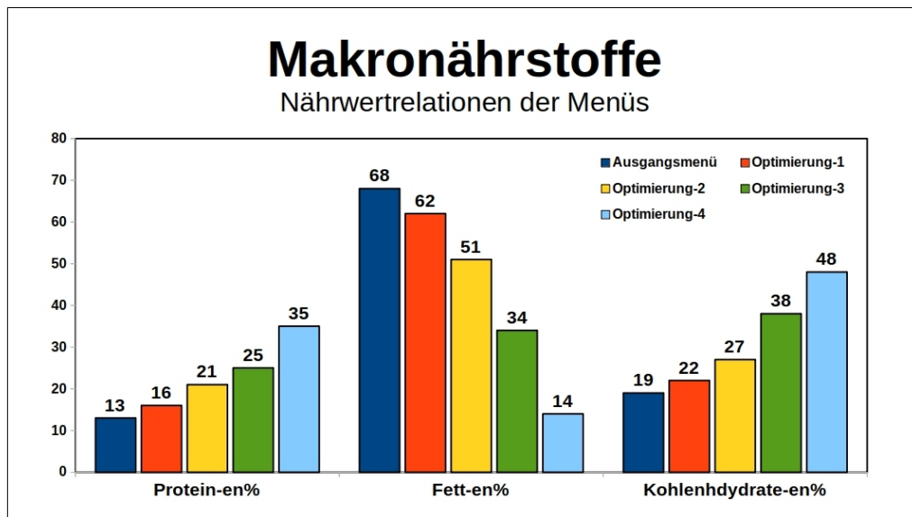
Abb. 6.2: Nährwertrelationen (en%=Anteil bezogen auf die Energie)
